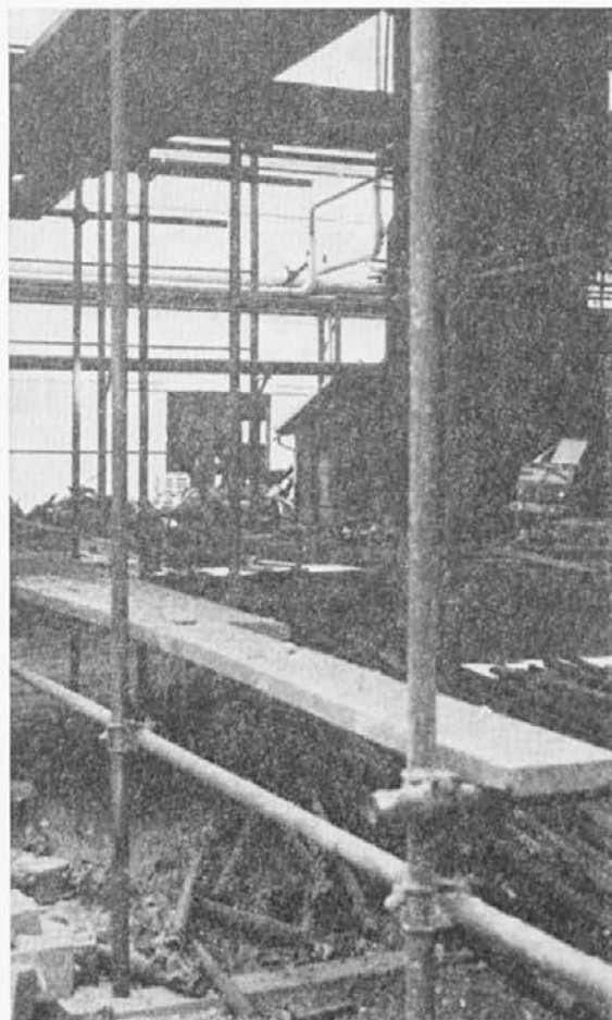
Delovni odri
