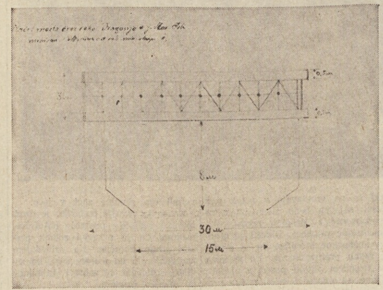
Načrt železniškega mostu čez reko Dragonjo pri Sečovljah v Istri. Odredovi minirajo most porušili v noči na 13. avgust 1944
