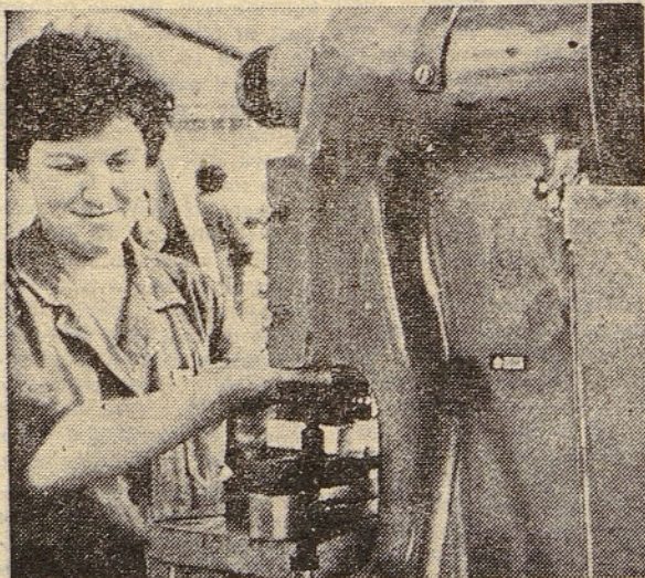
Tov. Angelca Štrbenk je zaposlena v proizvodnji avtomatskih telefonskih naprav. — Slika jo kaže pri delu na stikalnici, kjer štanca izolirne ploščice za ploščati rele
