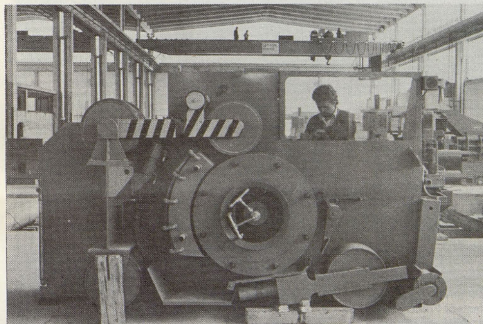
Montaža
