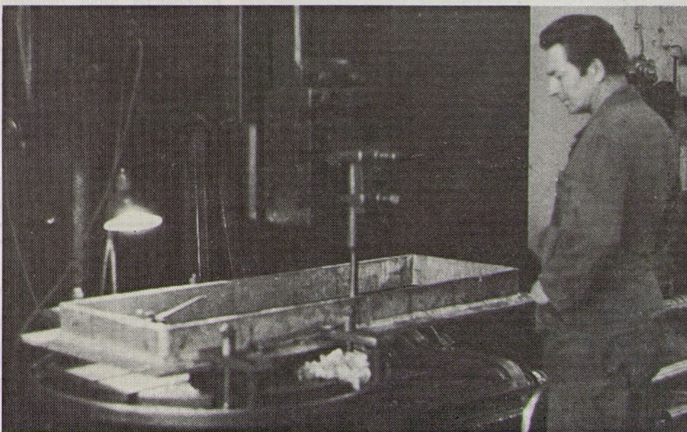
Izdelava kokile
