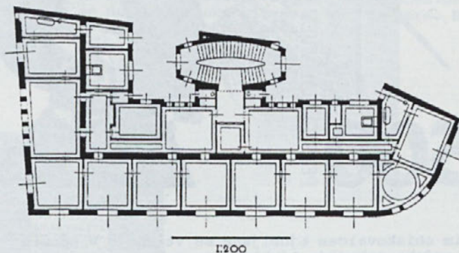
Zacherlova hiša na Dunaju, tloris (1903–1905)
