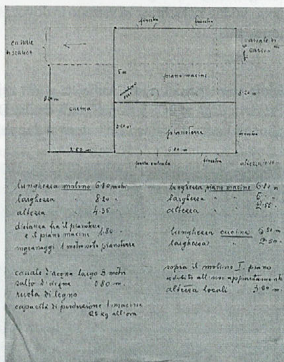
Skica mlina iz l.1937
