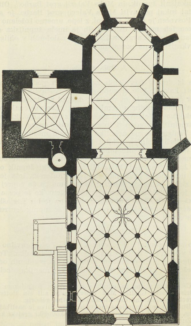
Tloris sedanje župnijske cerkve v št. Rupertu.
