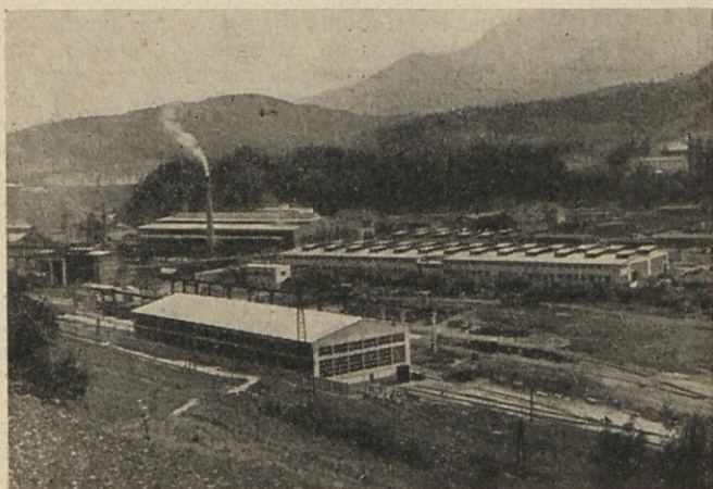
Obsežne naprave železarne v Ramah.
