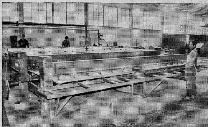
Lepljenje elementov za gradbene plošče
