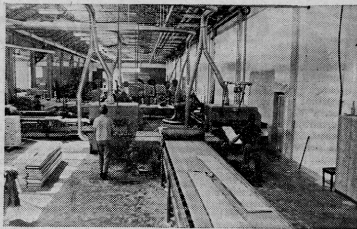
Širinski razrez žaganega lesa
