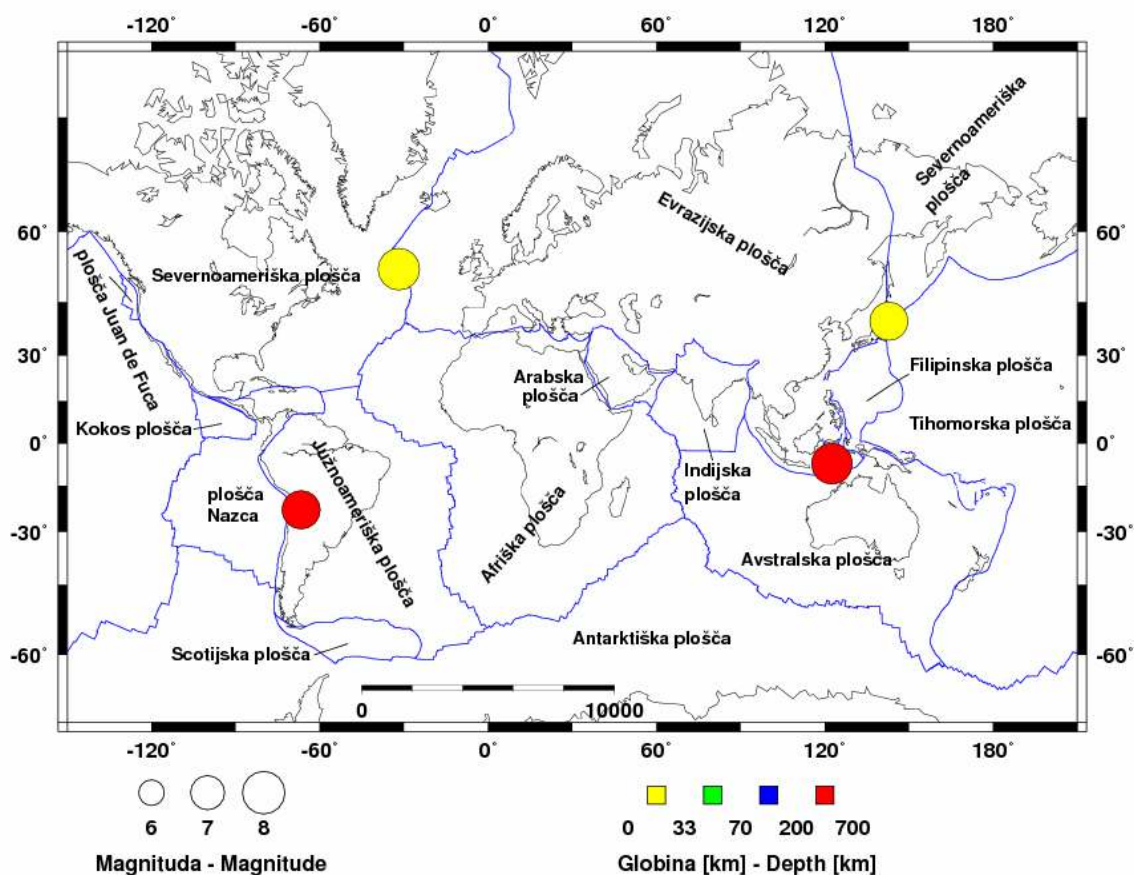
Slika 1. Najmočnejši svetovni potresi, februar 2015
