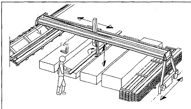
Slika 3: Mostna sortirno-zlagalna naprava
