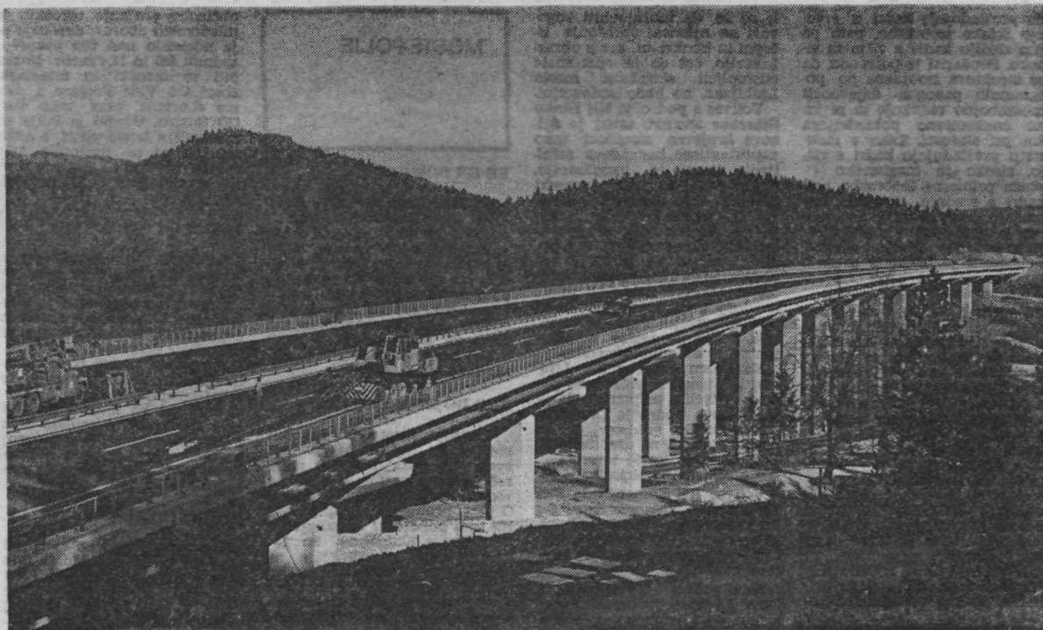
Viadukt »Ravbarkomanda« na odseku avtoceste Vrhnika — Postojna
