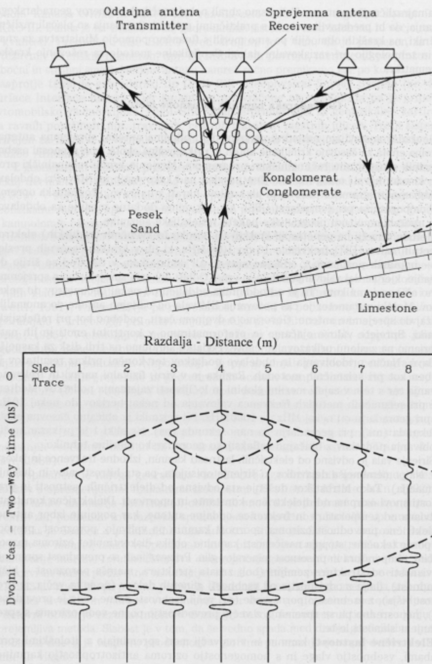
Sl. 1. Načelo georadarske meritve in rezultati v obliki radargrama
