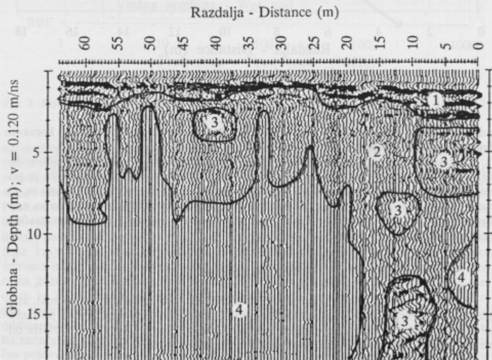
Sl. 5. Radargram iz kamnoloma Hotavlje
