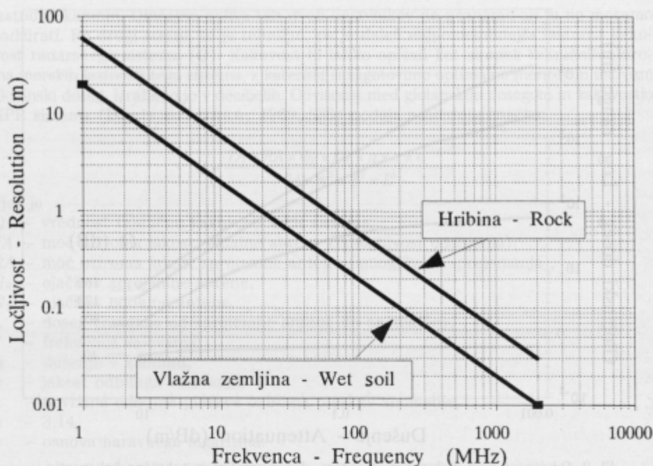
Sl. 3. Odvisnost ločljivosti od frekvence oddajne antene
