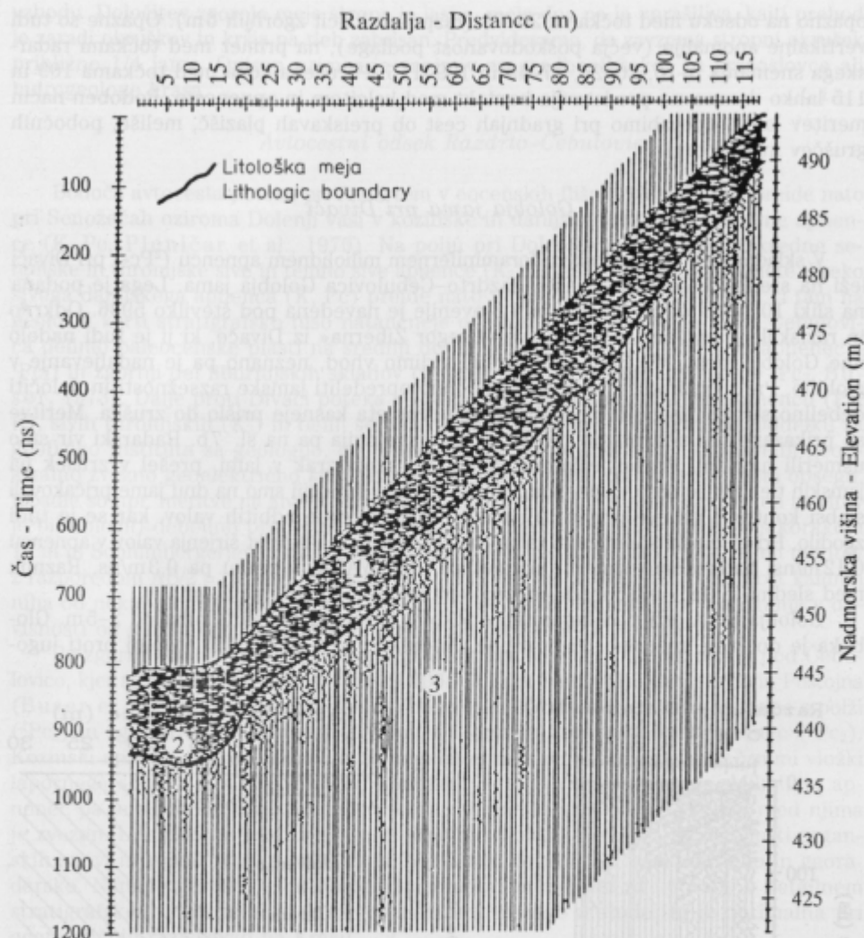
Sl. 6. Radargram iz kamnoloma Rudnika kalcita Stahovica 1 Pobočni grušč; 2 Aluvialni prod; 3 Kalcit – apnenec
