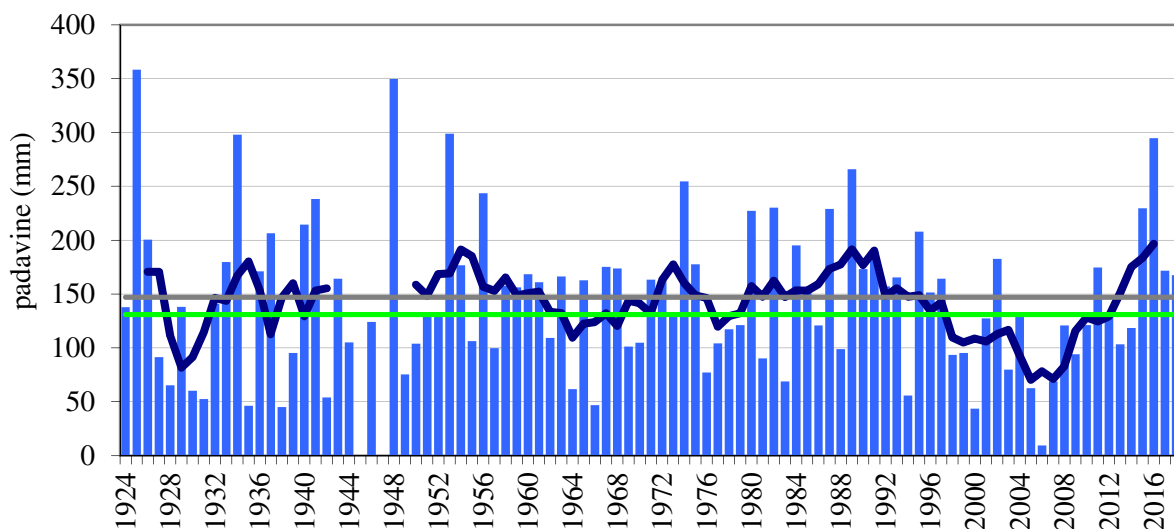
Slika 9. Junjska višina padavin (stolpci) in petletno drseče povprečje (krivulja) v obdobju 1924–2018 ter tridesetletni povprečji (1981–2010 zelena črta, 1961–1990 siva črta) v Zaloščah, razpoložljivi podatki
