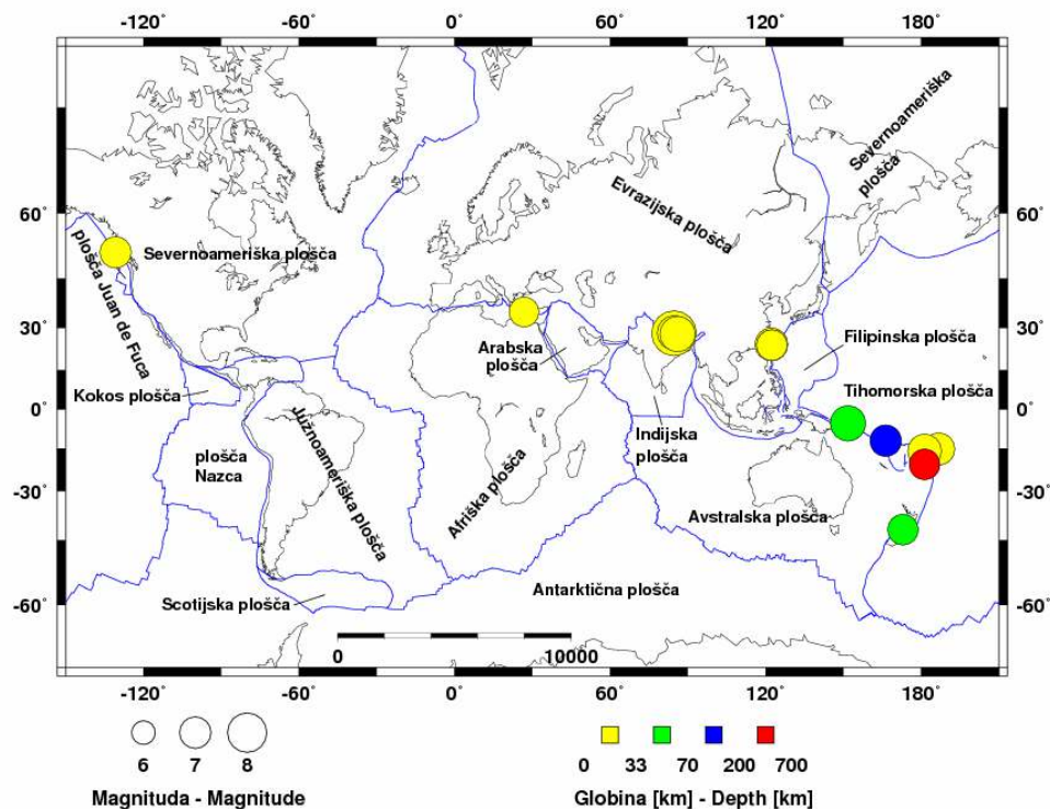
Slika 1. Najmočnejši svetovni potresi, april 2015 Figure 1. The world strongest earthquakes, April 2015
