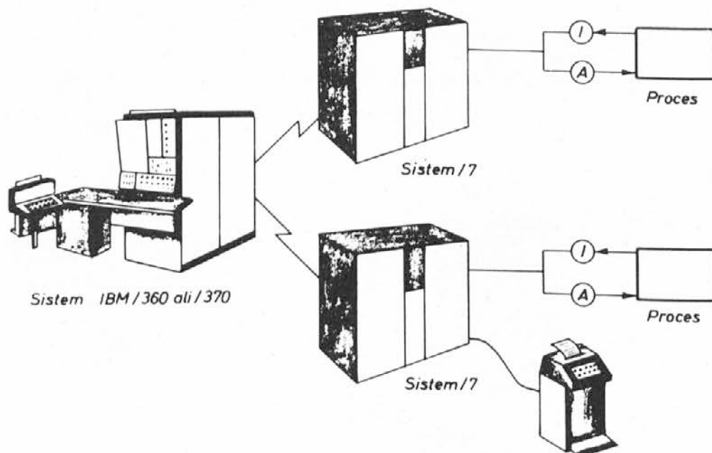
Sl. 2 Povezava procesnega računalnika IBM system/7 s centralnim računalnikom
