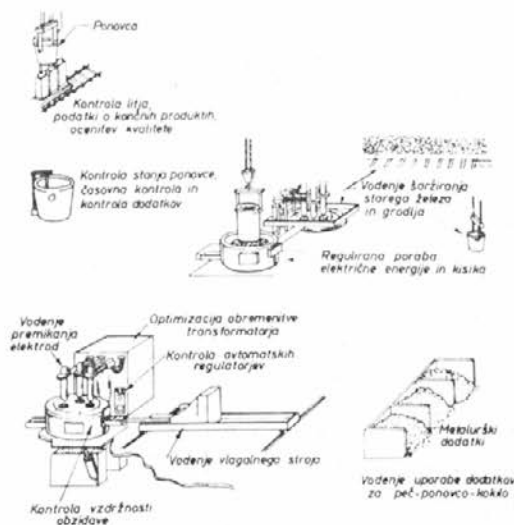
Sl. 1 Prikaz uporabe procesnega računalnika pri delu elektroobločne peči
