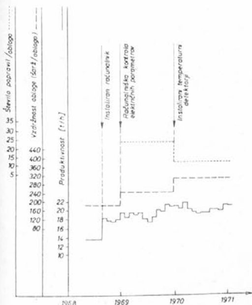
Sl. 5 Produktivnost peči in vzdržnost obloge pri računalniško vodenih elektroobločnih peči
