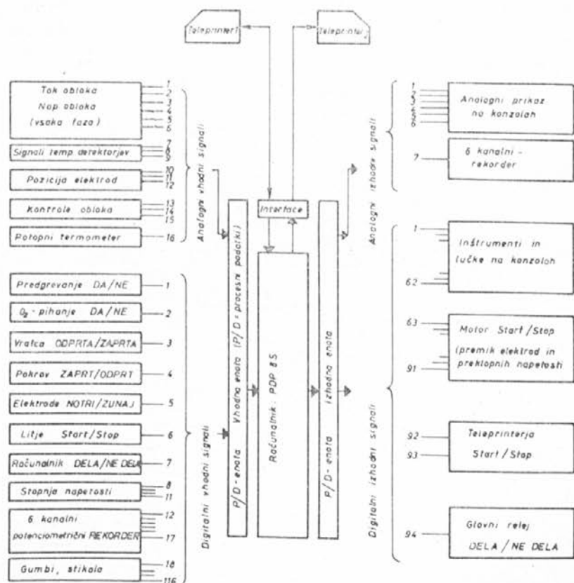
Sl. 4 Računalnik z vhodnimi in izhodnimi signali 12,13
