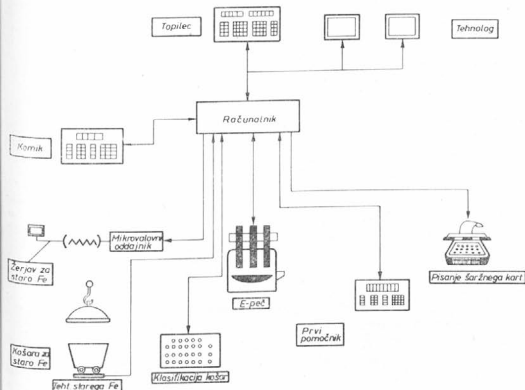
Sl. 3 Sistem povezave elementov računalniško vodenega procesa
