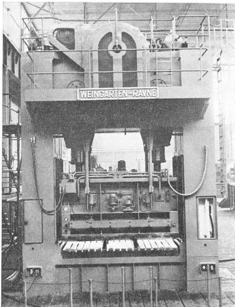
Slika 1 — ekscentrična dvostebna stiskalnica DQ 500, namenjena za hladno plastično preoblikovanje
