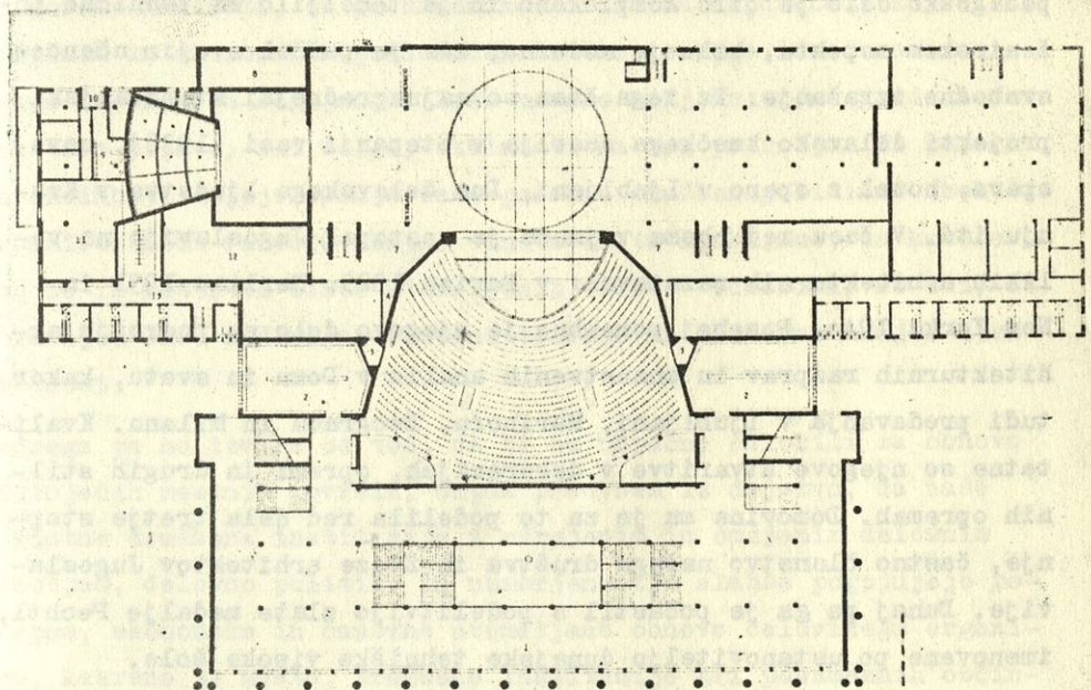
Ivan Vurnik: Opera na trgu Revolucije, projekt, 1952
