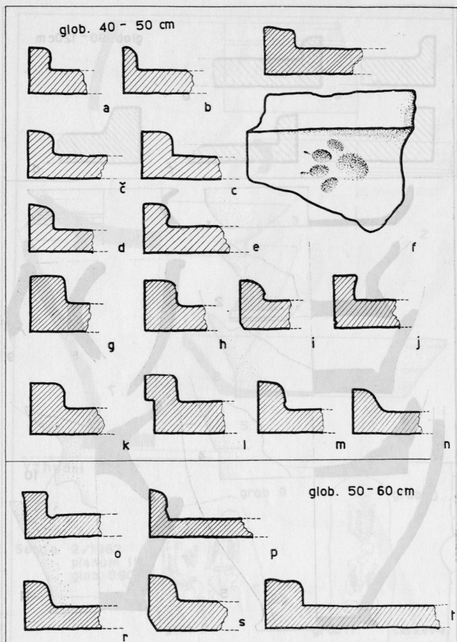
Tegule iz globine 40—60 cm. Na fragmentirani opeki f je znamenje volčje šape. Vse 1 : 4 (risala J. Šubert)
