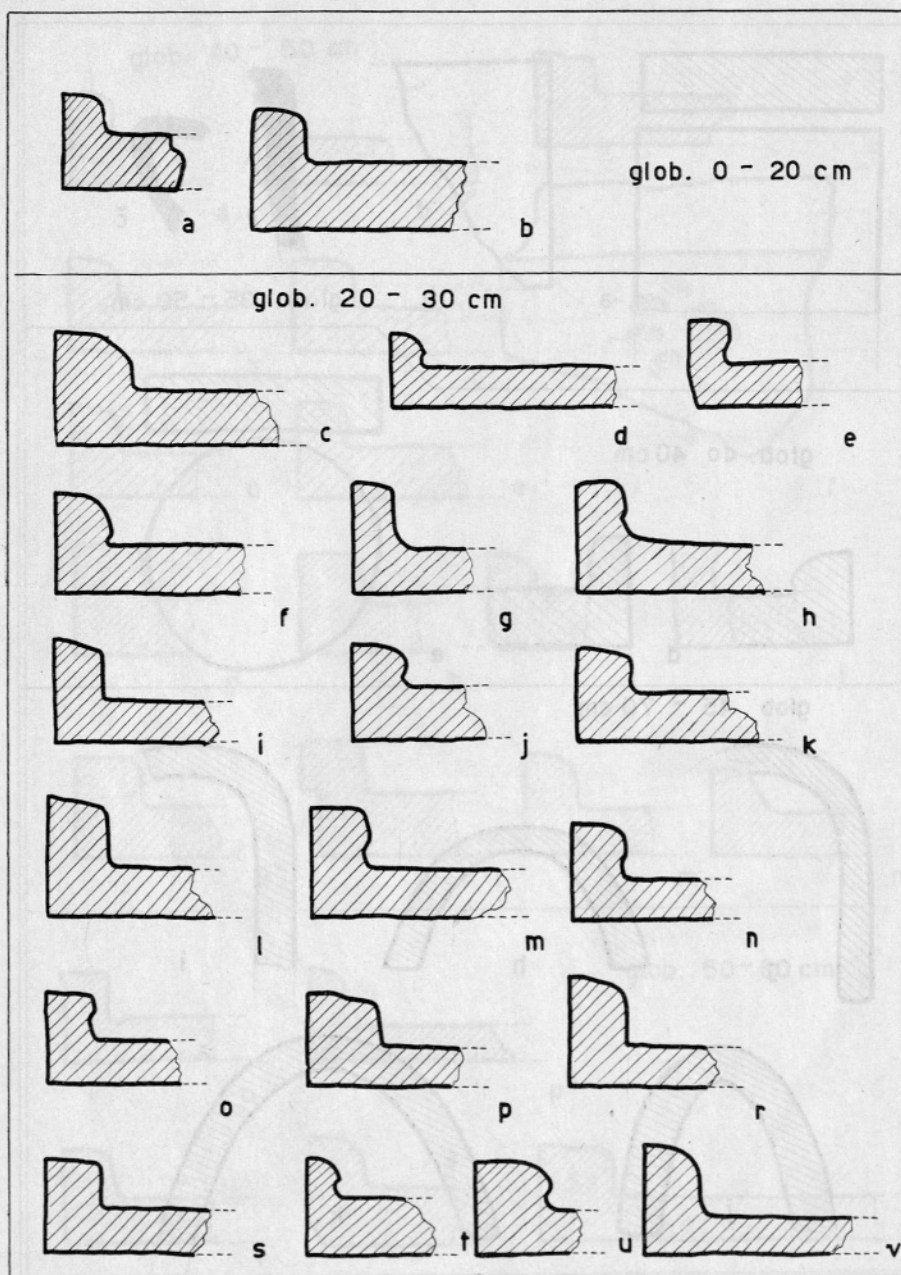
Velika vas, tipi tegul iz kvadrantov, sortirani po globini. Vse 1 : 4 (risala J. Šubert)
