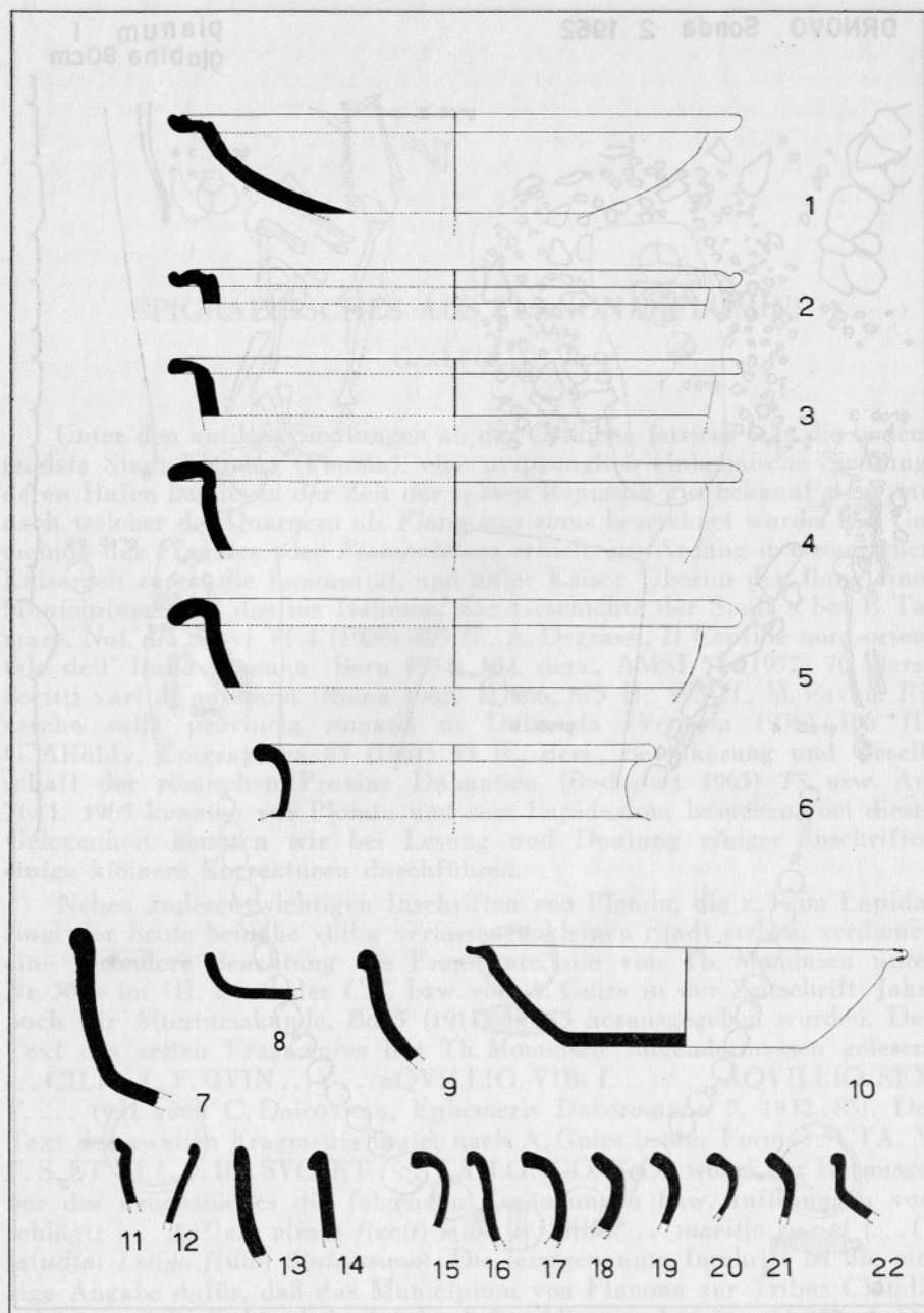
Drnovo, lončarska peč na parc. 90/6, izbor karakterističnih profilov skodel. Vse 1 : 4 (risala J. Šubert)
