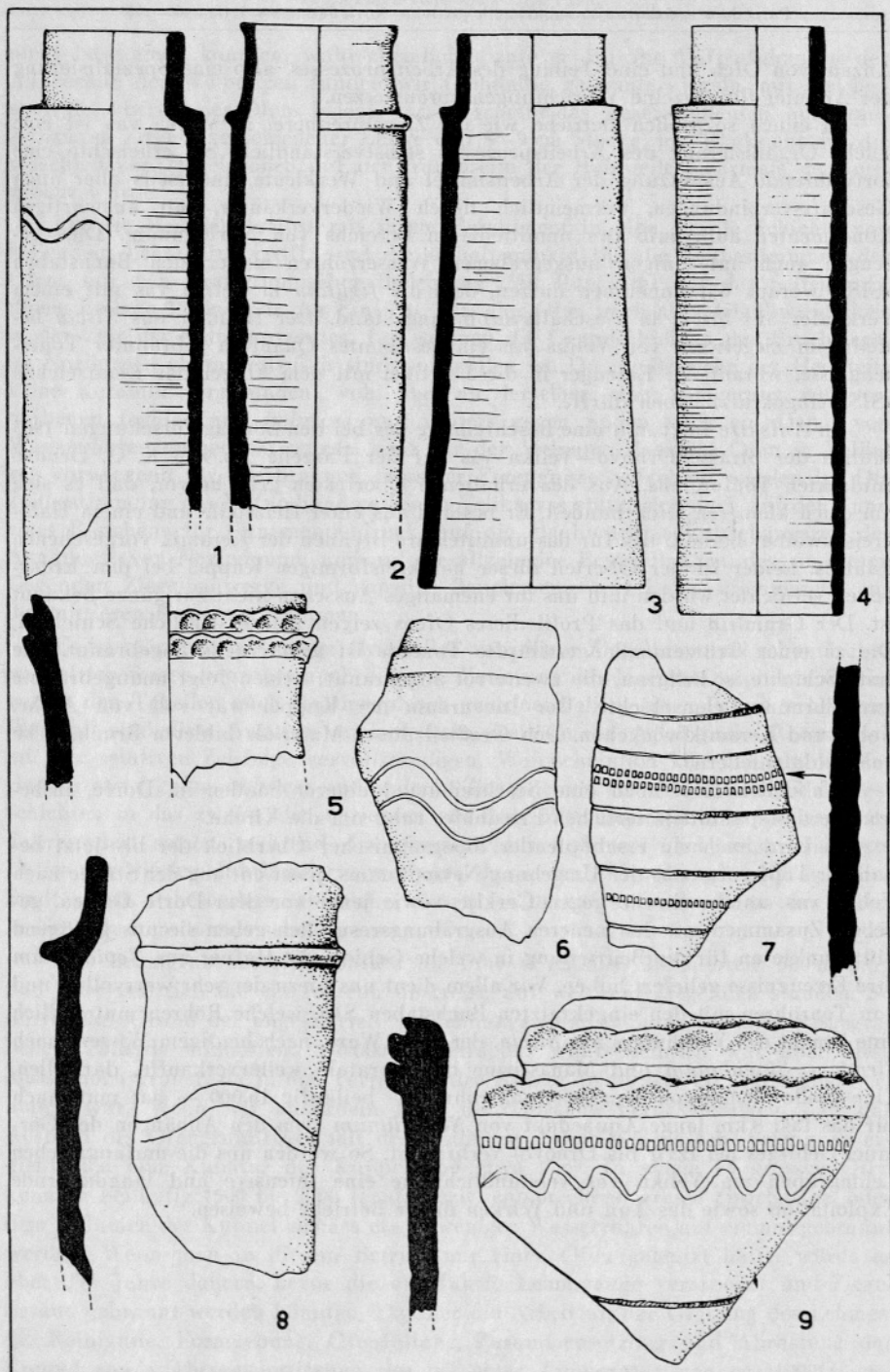
Velika vas, primerki okrašenih in neokrašenih vodovodnih cevi z južnega dela jarka B. 1—4 = 1 : 8; 5 = 1 : 4, ostalo 1 : 2 (risala J. Subert)
