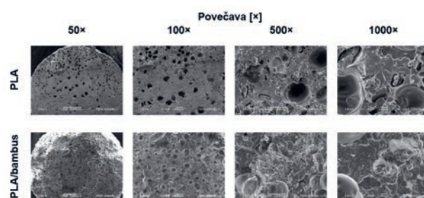
Slika 2: Prečni prerez PLA in PLA/bambus filamentov
