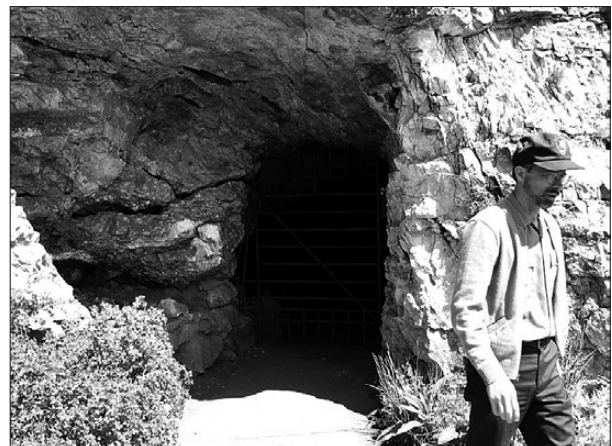
Fig. 9: Historic Entrance of Jewel Cave, South Dakota (USA) (Photo: A. Pflitsch).
