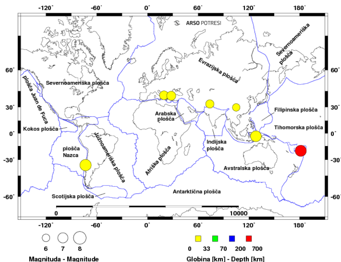
Slika 1. Najmočnejši svetovni potresi, september 2019
