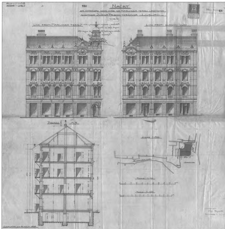
16 Stanovanjsko-trgovska stavba na Prešernovem trgu 3 in Čopovi ulici 1, 1896, fasadi, prerez, situacija, gradnja, kolorirana kopija / 56,5 x 58; ZAL, Načrti (LJU 334), Restavrirani in konservirani načrti, R-004-24
