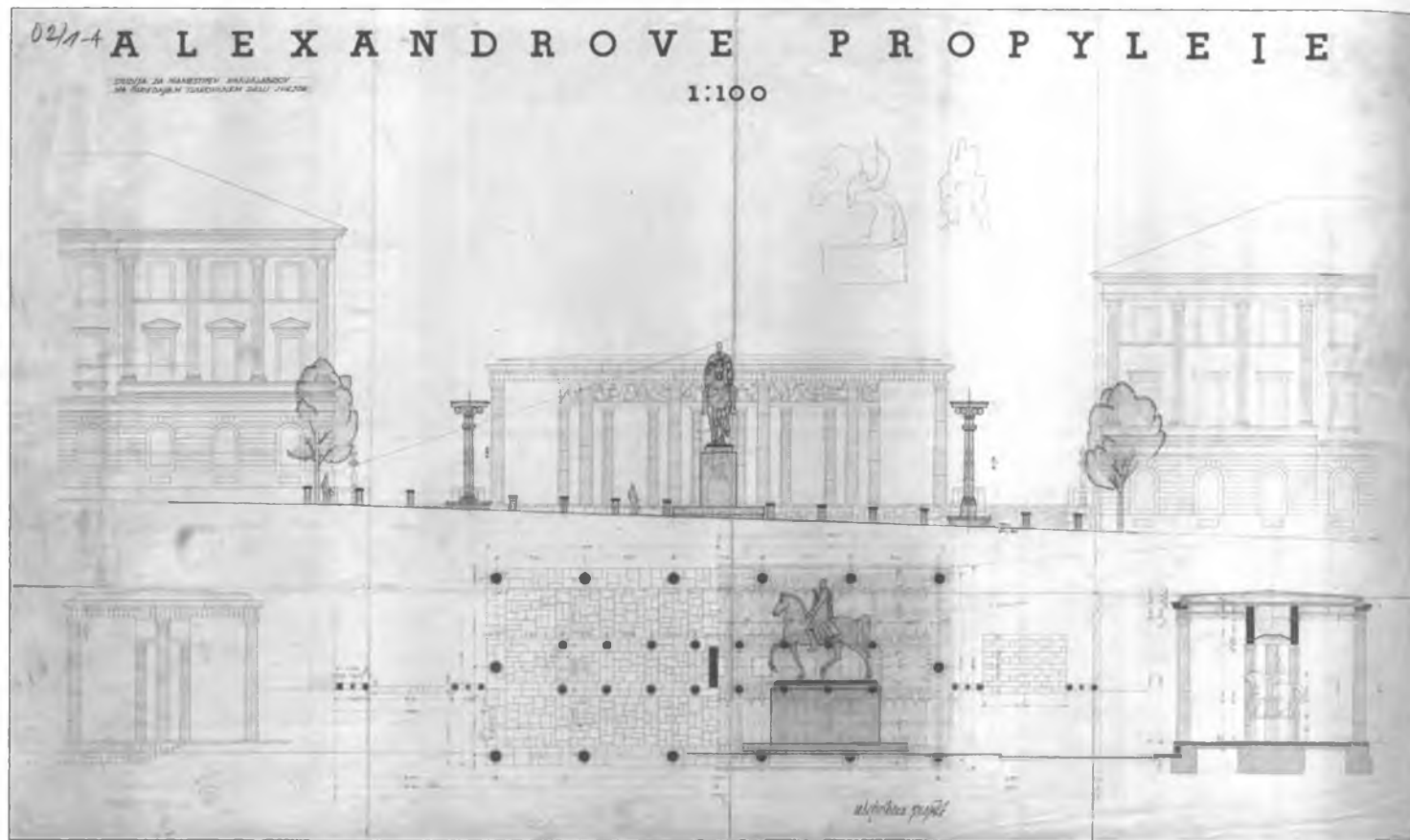
13 Jože Plečnik in Boris Kobe, Ureditev za namestitvev kandelabrov na osrednjem tlakovanem delu Zvezde, postavitvev Aleksandrovega spomenika in propilej na Južnem trgu, 1936 in 1940, pogleda, tlorisa in prereza, kolorirana kopija z originalnimi popravki arh. Kobeta / 82,8 x 48,8; ZAL, Načrti (LJU 334), mapa 002-001-03
