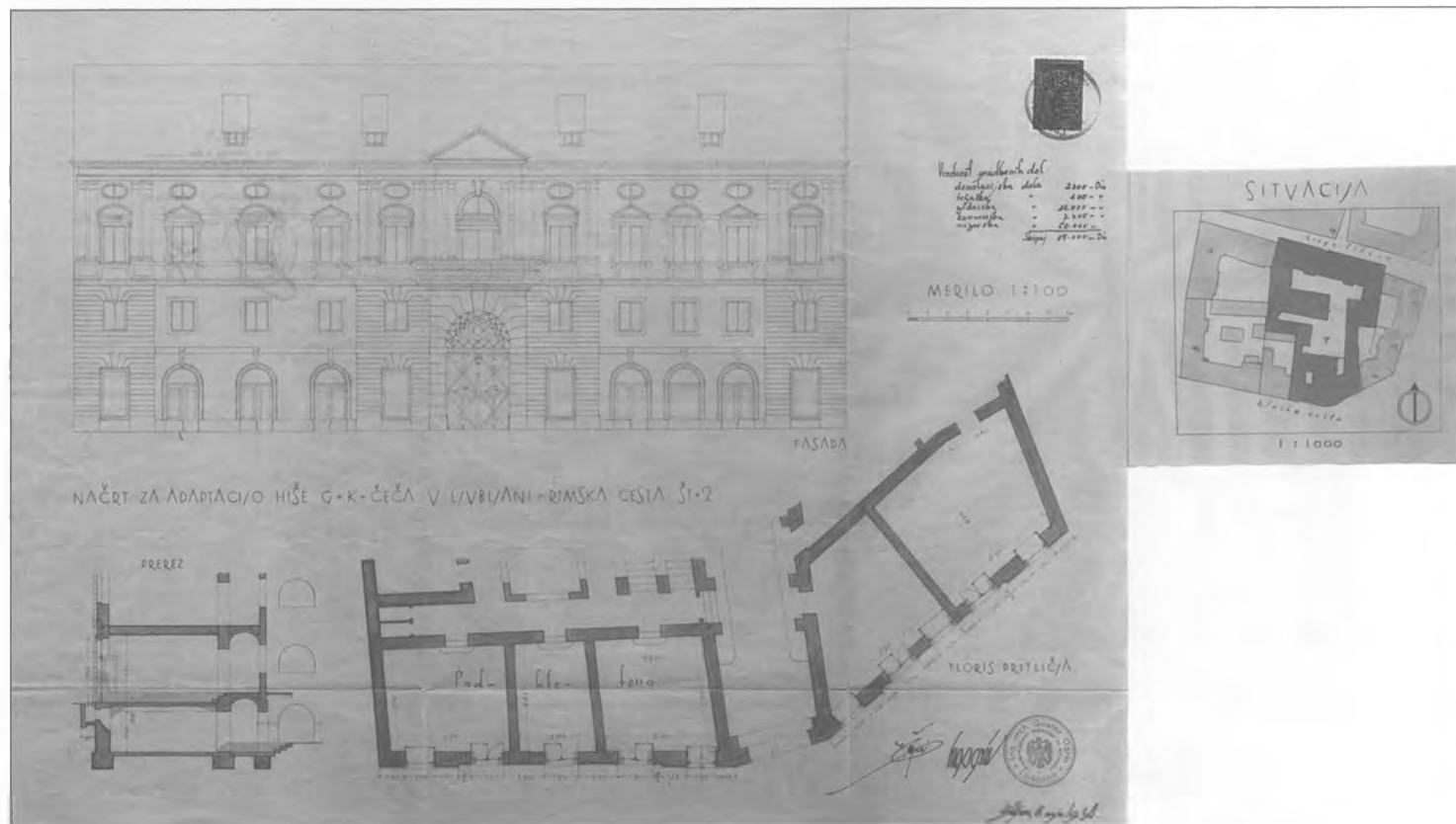
20 Stanovanjska hiša na Rimski cesti 2, 1934, glavna fasada, prerez, tloris pritličja in situacija, adaptacija, kolorirana kopija / 74,4 x 41,1; ZAL, Mesto Ljubljana, gradbena registratura (LJU 493), Reg IV
