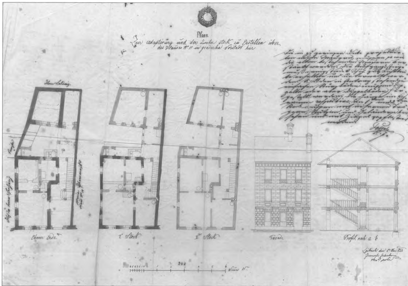
19 Stanovanjska hiša v Gregorčičevi ulici 10, 1854, tlorisi pritličja, 1. in 2. nadstropja, glavna fasada in prerez, adaptacija in gradnja 2. nadstropja prizidka, kolorirana matrica / 59,2 x 41,1; ZAL, Mesto Ljubljana, splošna mestna registratura (LJU 489), Reg I, sv. 7, f. 508
