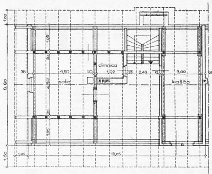
Tloris podstrešja istega doma.
