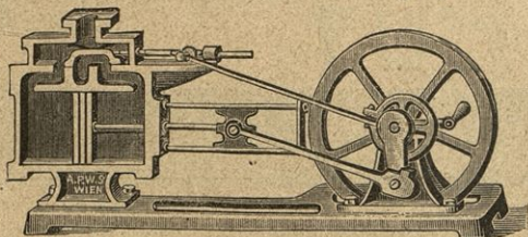
692 Durchschnittsmodell des Dampfzylinders.
