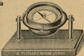
698. Kompas za ladje.
