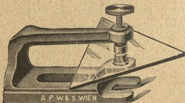
650. Klangfigurenapparat.
