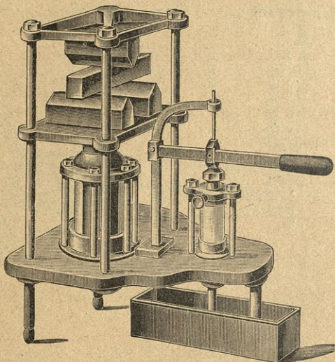
626. Hydraul. tiskalo.
