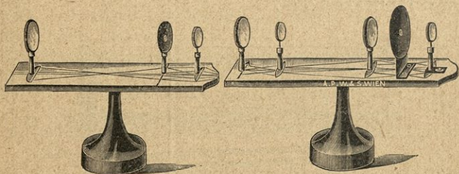
671. Drobnogled.
