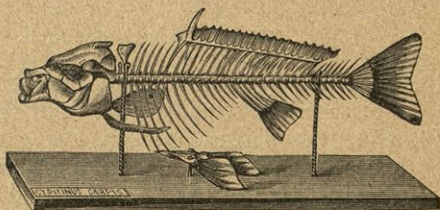
516. Karpfen-Skelett.
