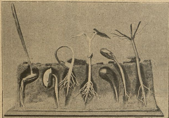
517. Keimungsmodell.
