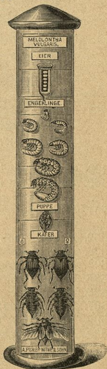
495. Rjavi hrošč.
