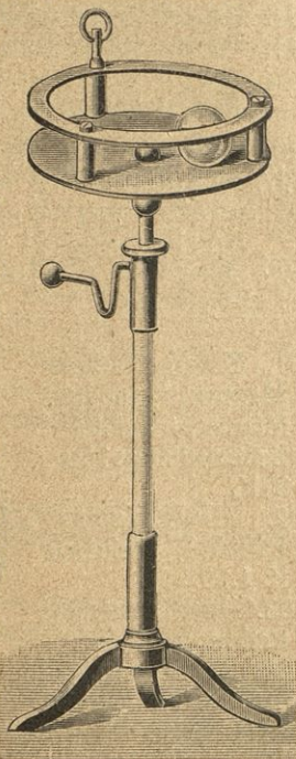
714. Kugellauf (Nebenapparat für Influenzmaschine).
