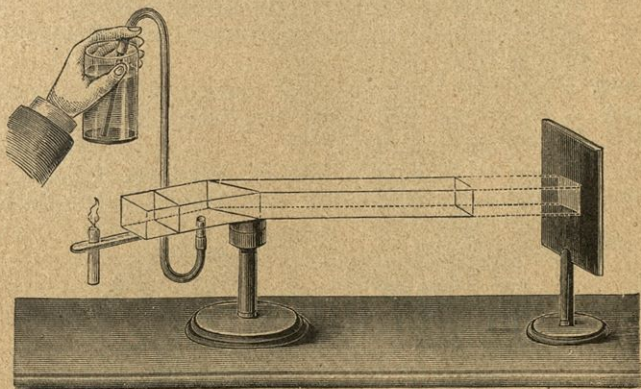
677. Lichtbrechungsrinne nach Neumann.
