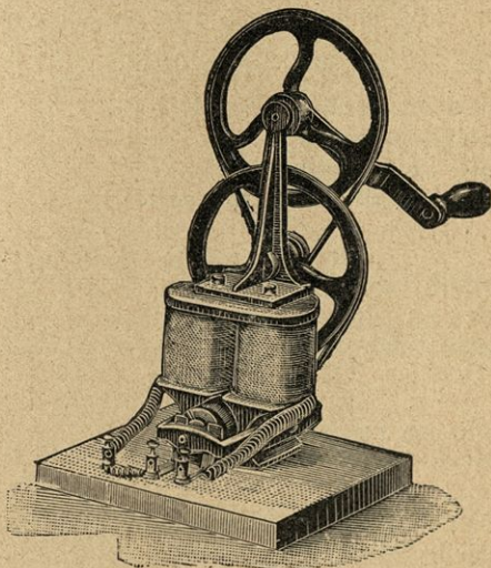
732. Dynamo-stroj.
