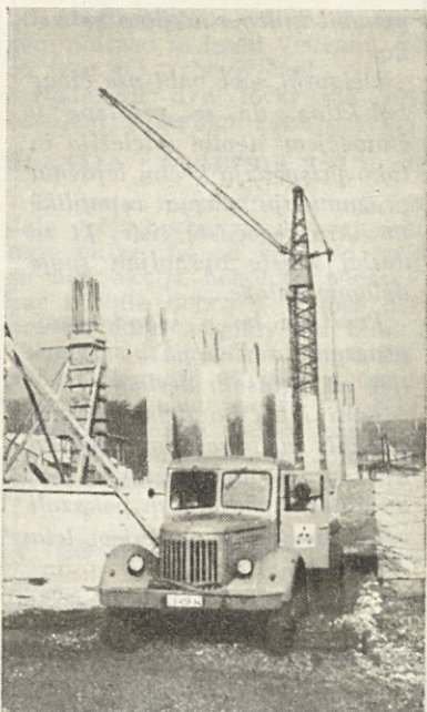
Temelji in prvi oporni stebri za stavbo premaznega stroja
