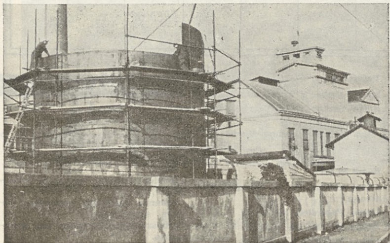
Gradnja posode za tekoče gorivo ob kotlarni na Vevčah
