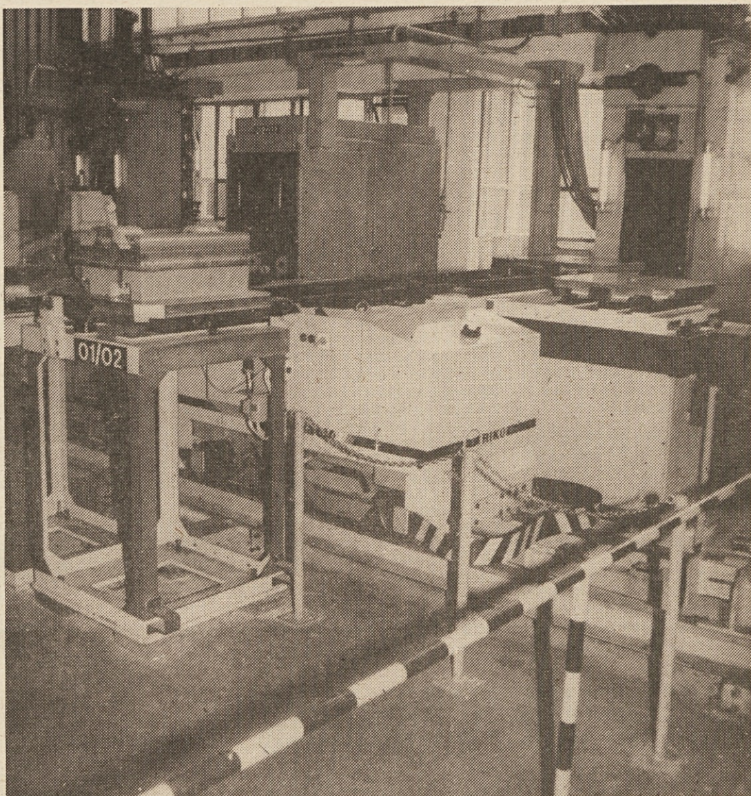
Avtomatski transportni voziček, postavljen v Prvomajski Zagreb, kjer oskrbuje obdelovalno linijo. Na 32. mednarodnem beograjskem sejmu nove tehnologije in fleksibilne avtomatizacije v industriji – Integra 88 je prejel Rikovo Avtomatski transportni voziček ta 630 Zlato plaketo za vrhunski prodor jugoslovanske industrije na področju nove tehnologije in fleksibilne avtomatizacije v industriji.
