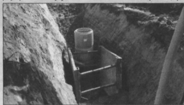
Polaganje cevi med Drožanjskim in Florjanskim potokom na kanalu A (foto: arhiv Občine)
