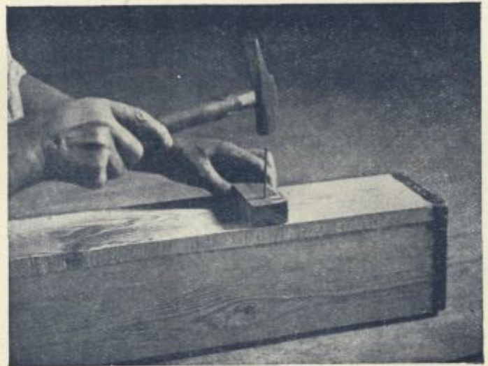
Na zaboječek pribijemo lesene količe.
