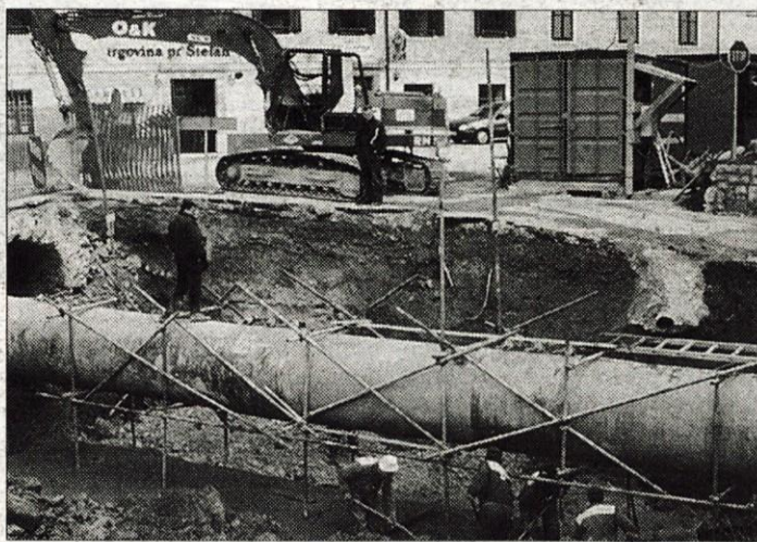
Sledi Selc je velika gradbena jama, v kateri pripravljajo temelje za novi most. Selnica teče začasno po veliki železni cevi.
