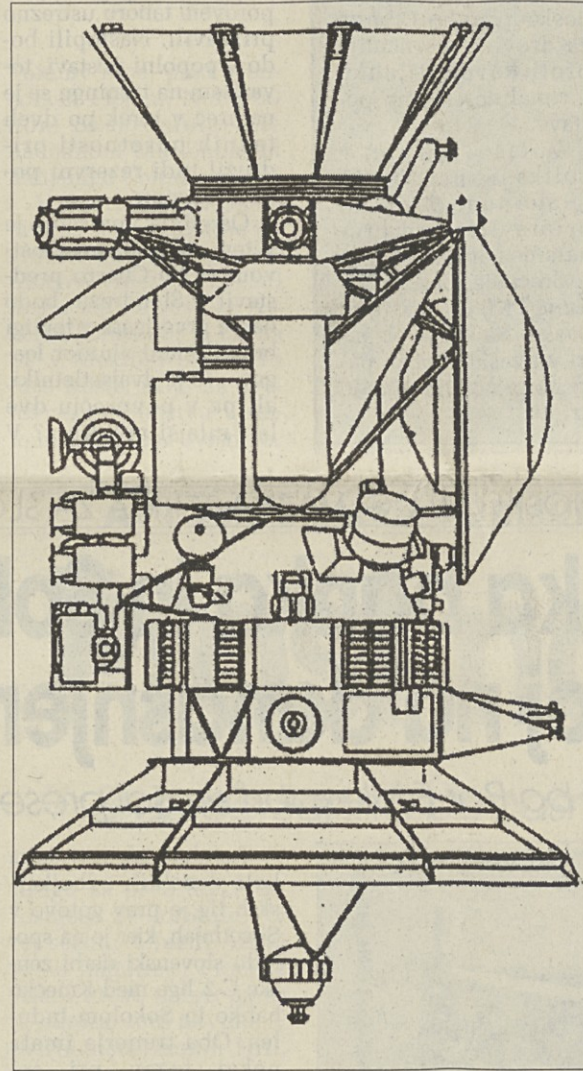
Sedanja zasnova sonde za polet proti Plutonu, ki ima močno zmanjšano maso.
