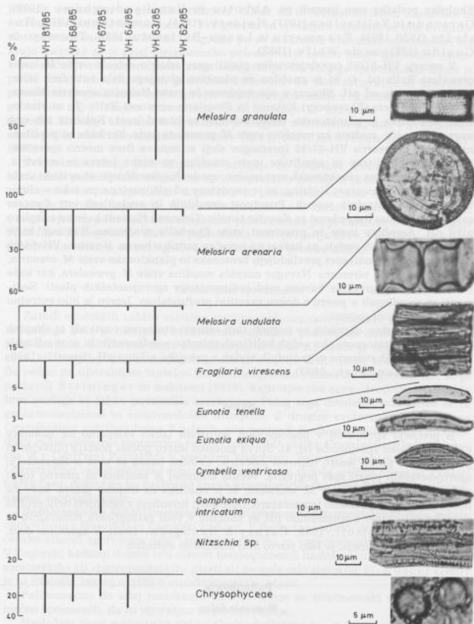
Sl. 4. Vertikalna razporeditev relativne gostote najpomembnejših vrst diatomej
