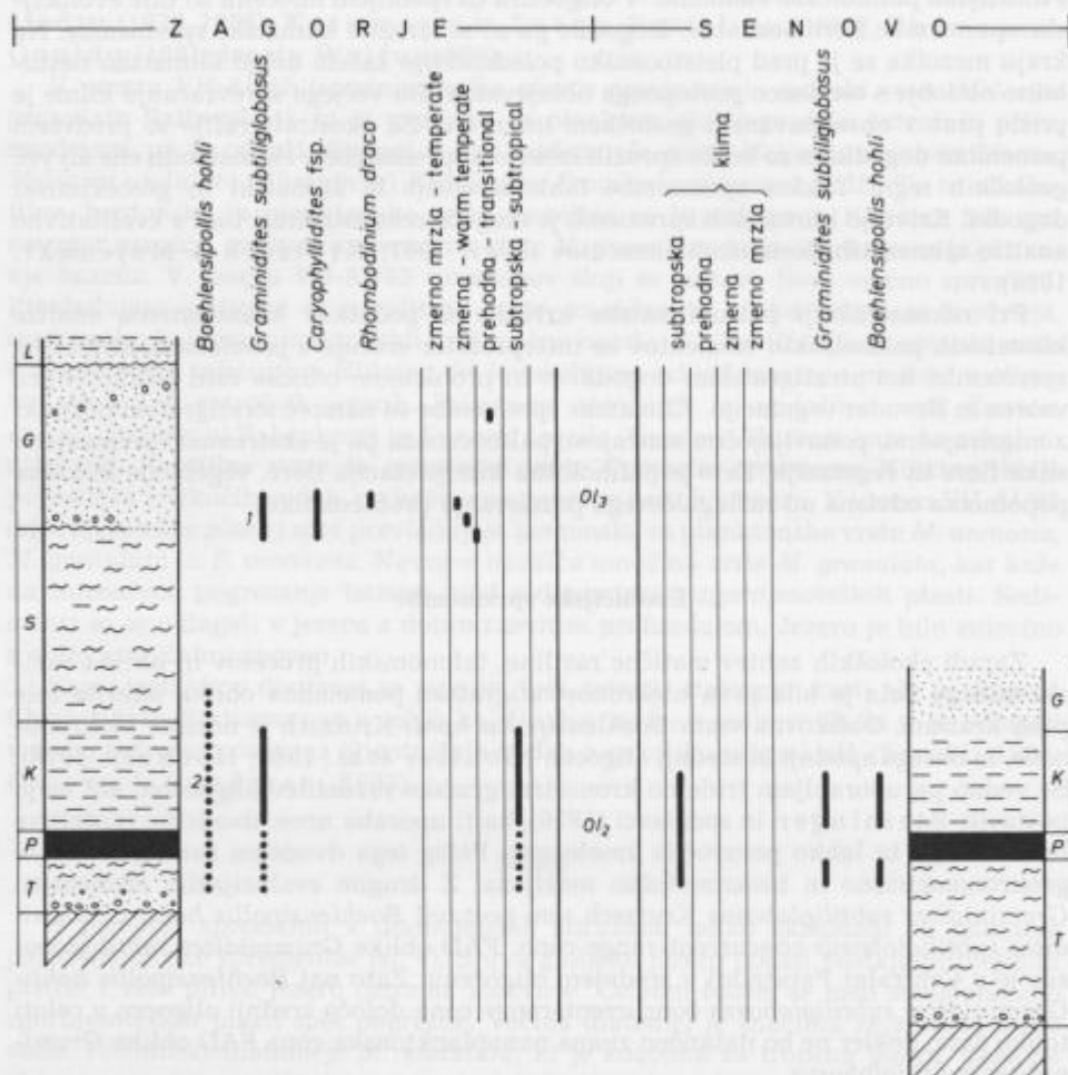
Sl. 5. Kronostratigrafski položaj »soteskih« in »govških« plasti v Zagorju in Senovem po razpoložljivih palinoloških podatkih. Litostratigrafska stolpca po Placerju (1984) in Uhanu (1986)
