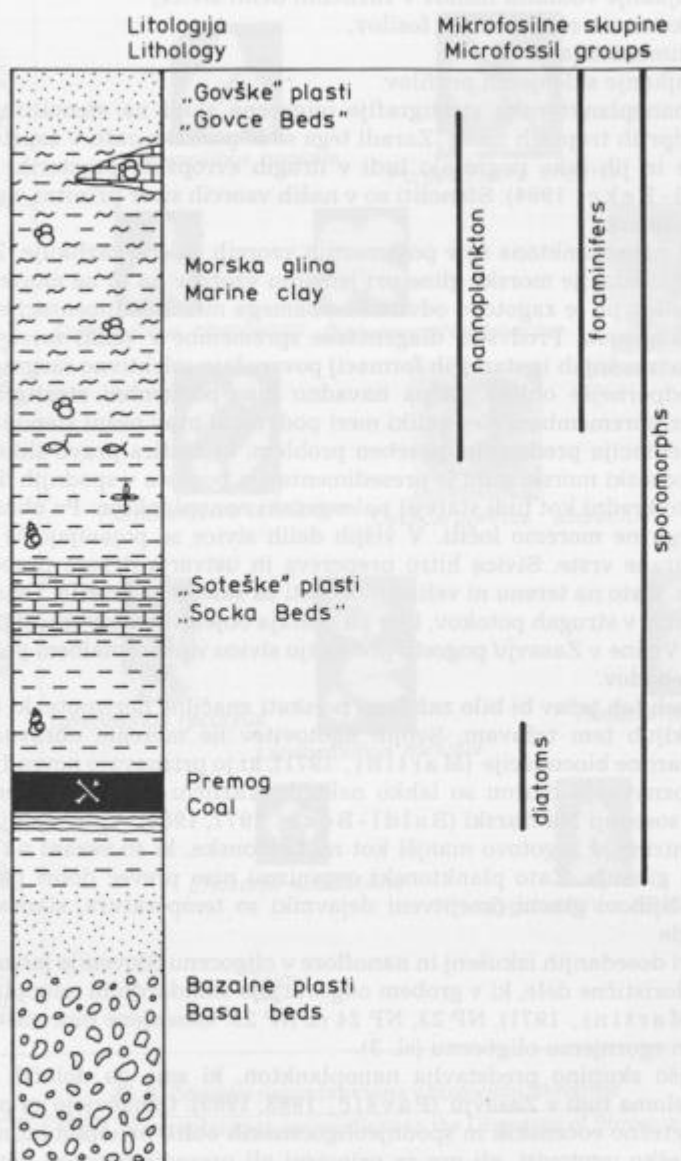
Sl. 2. Porazdelitev mikrofosilnih skupin v oligocenu Zasavja.
