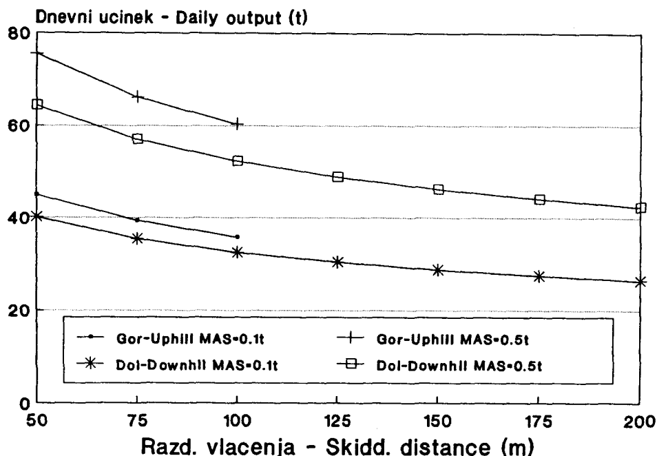
Slika 5 Primerjava dnevnih učinkov spravila lesa navzgor in navzdol
