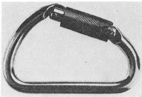
Na sliki je vponka tipa TL (Twist Lock) firme Elite. Skoraj vse firme, ki v Evropi izdelujejo vponke, ponujajo zdaj vsaka svojo varianto novega tipa vponke
