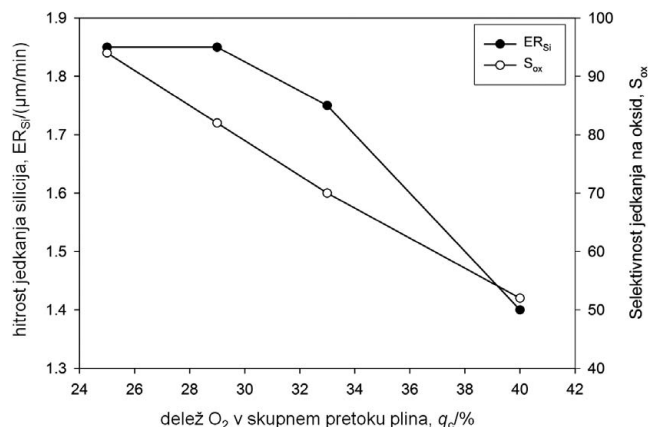
Slika 3: Hitrost jedkanja silicija in selektivnost jedkanja oksidne maske v odvisnosti od deleža \text{O}_2 v skupnem pretoku plina
