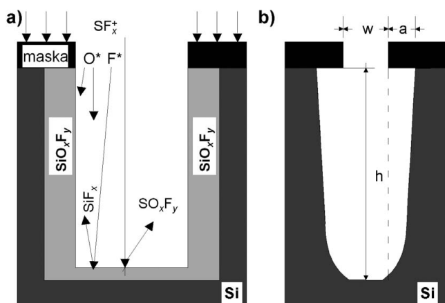
Slika 2: Shematski prikaz mehanizma usmerjenega jedkanja z RIE in \text{SF}_6/\text{O}_2 -kemijo: a) idealni usmerjeni profil in b) realni profil s prikazanim lateralnim spodjedkavanjem a in pozitivnim nagibom stranskih sten profila globine h ter širine odprtine w .
