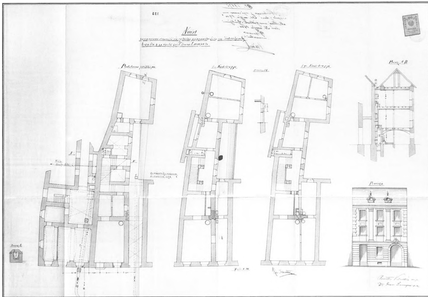
28 Stanovanjska hiša dr. Franca Lampeta na Ciril-Metodovem trgu 4, 1900, tlorisi etaž, prerezi, fasada, adaptacija, matrica / 75,1 x 51,7, ZAL, Mesto Ljubljana, splošna mestna registratura (LJU 489), Reg I, f. 1155, fol. 333
