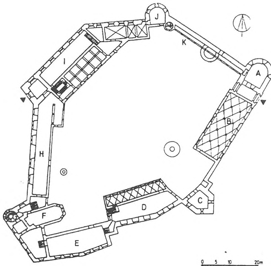
Grajski tloris. Priredil I. Gričar.
