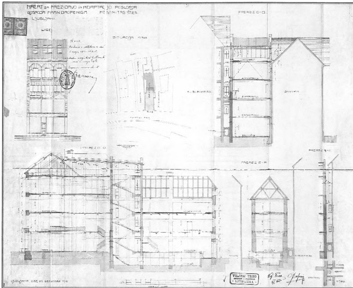
35 Trgovska hiša Franca Drogeniga na Mestnem trgu 23, 1914, fasada, situacija in prerezi, adaptacija, matrica / 72,6 x 57,8, ZAL, Mesto Ljubljana, splošna mestna registratura (LJU 489), Reg I, f. 1790
