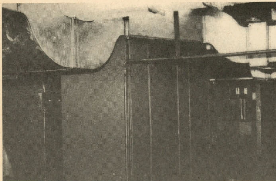
Pogled na pogonsko postrojenje za zračno hlajenje enot v strojnem centru Informatike, Velenje
