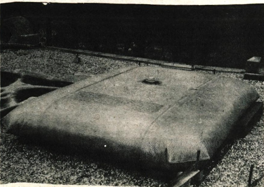
Tri leta je gumijasti rezervoar za vodo že izpostavljen dežju in soncu. Razpoke nima še prav nobene.
