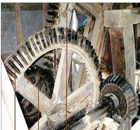
bak veliko zobato kolo ploščati prenos (lesen) ploščati prenos (železen)
