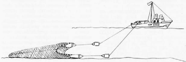
POVLEČNA GLOBINSKA MREŽA — obstajajo različne mreže za ulov na trdem, peščenem ali blatnem morskem dnu
