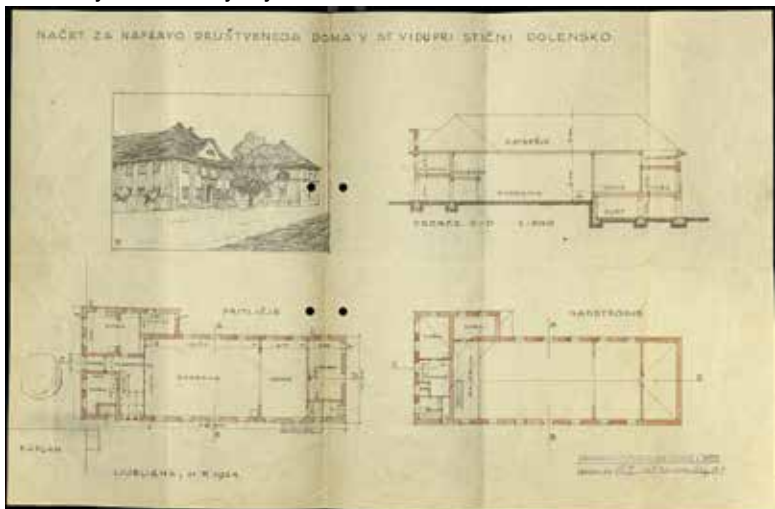
Načrt za gradnjo Katoliškega prosvetnega doma v Šentvidu pri Stični. Načrt hrani Nadškofijski arhiv v Ljubljani.
