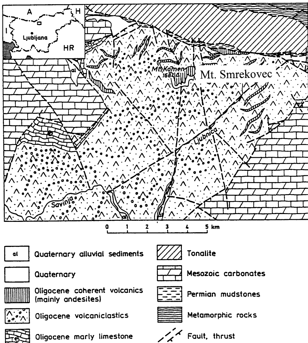
Figure 1. Simplified geological map of the Smrekovec volcanic complex (after Mioč, 1983) Slika 1. Poenostavljena geološka karta Smrekovškega vulkanskega kompleksa (po Mioču, 1983)
