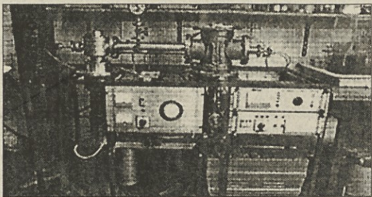
Visokovakuumski naparovalnik ogljika C 60 .
