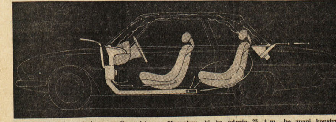
Na mednarodni razstavi prevoznih sredstev v Muenchnu, ki bo odprta 25. t.m., bo znani konstruktor Pininfarina razstavil svoj model »PF Sigma« kot najbolj varno vozilo. Na sliki »Sigma« v prezezu
