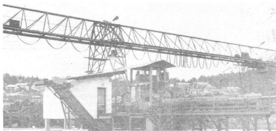
Nova naprava - kakovostno obdelana in razrezana hlodovina - Hojina Žaga na Škofljici je z novo naložbo začela lansko jesen. Linija za razrez lesa je stala 85 milijonov. Ob njej bosta dovolj dva človeka, saj je naprava avtomatska in računalniško vodena.
