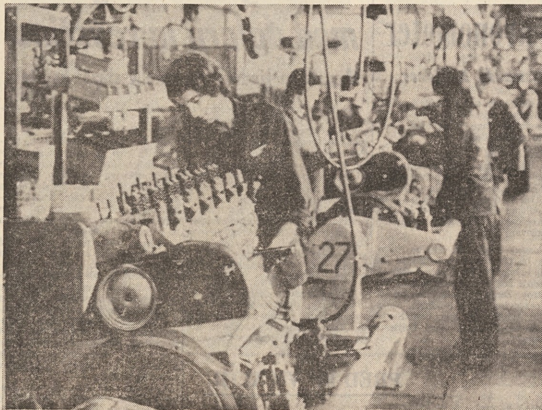
V sarajevski tovarni Famos so pred nedavnim na osnovi sporazuma z zahodnonemško tovarno Daimler-Benz začeli proizvajati znane mercedesove motorje za teška vozila. Na sliki: montažni trak tovarne.
