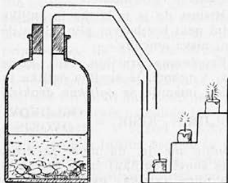
Ogljikov dvokis je težji od zraka in preprečuje gorenje
