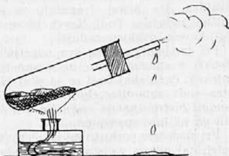
Če sladkor segrevamo v zaprti posodi, uhaja plin in uhaja tekočina, v posodi ostane pa ogljik
