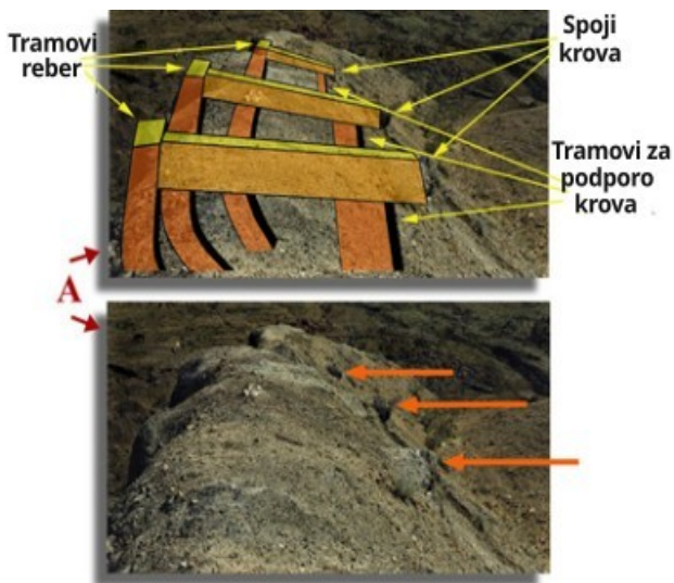
Slika 44: Rebra in nosilci krova.
