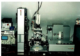
Slika 201: Mikroskop v sedanjem »izboljšanem« stanju.
