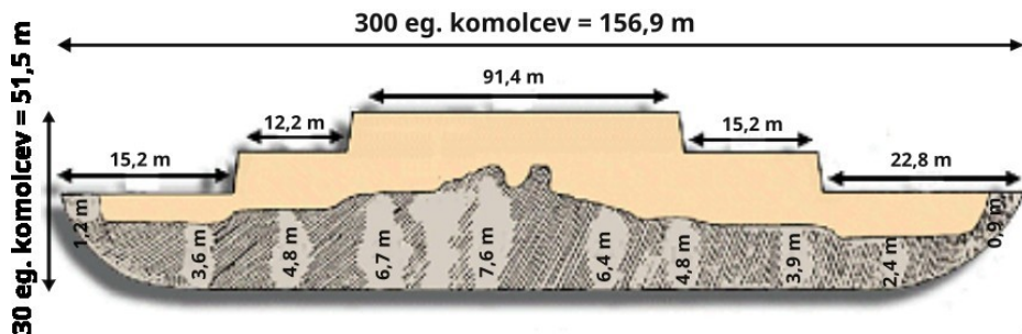
Slika 10: Biblijske dimenzije ladje.
