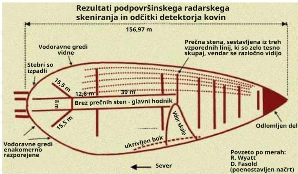
Slika 8: Ugotovljene notranje dimenzije in struktura objekta.
