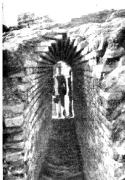
Slika 62: Obokana drenaža, še vedno vodoodporna.
