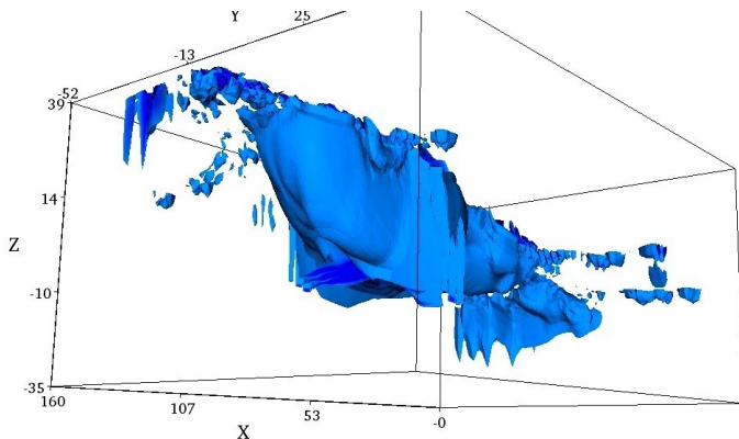
Slika 16: Skeniranje zemlje pod ladjo.
