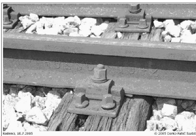
Slika 13: Tirnica, vgrajena leta 1942, je še vedno vgrajena na progi Ljutomer–Gornja Radgona in po njej poteka promet vlakov s hitrostjo do 60 km/h.
