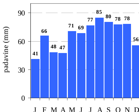
Slika 8. Dnevna najvišja višina padavin po mesecih v obdobju 1949–junij 2015 na Strojni
