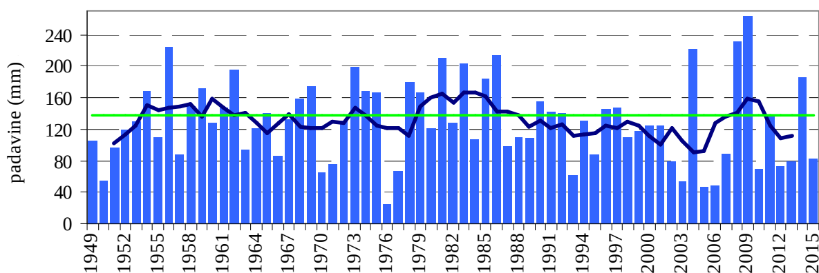
Slika 6. Junjska višina padavin (stolpci) in petletno drseče povprečje (krivulja) v obdobju 1949–2015 ter referenčno povprečje (zelena črta) na Strojni
