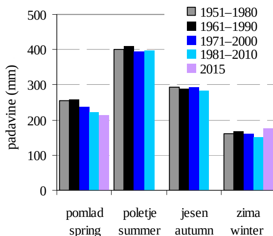
Slika 4. Povprečna višina padavin po letnih časih in po obdobjih ter v letu 2015 na Strojni; zima 2014/15
