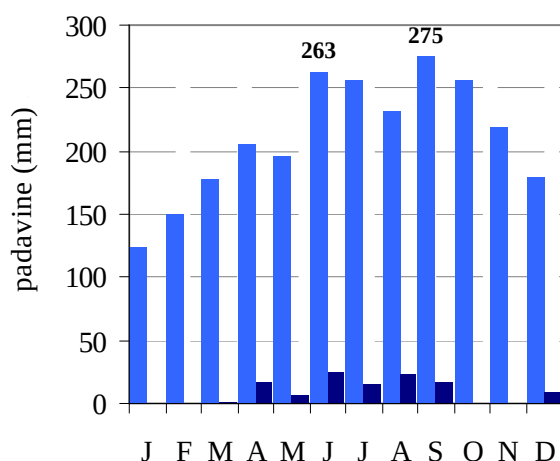
Slika 7. Mesečna najvišja in najnižja višina padavin v obdobju 1949–junij 2015 na Strojni
