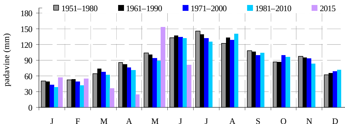
Slika 5. Mesečna povprečna višina padavin po obdobjih in izmerjena leta 2015 na Strojni
