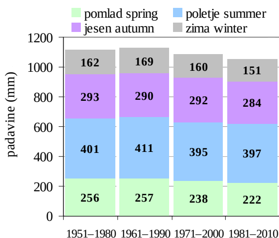
Slika 3. Povprečna višina padavin po obdobjih in po letnih časih na Strojni
