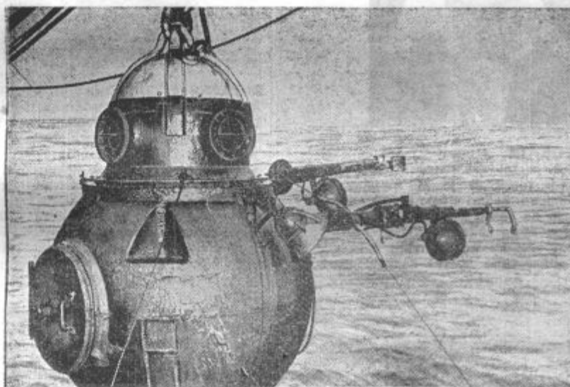
POTAPLJAŠKI ZVON Z ROKAMI. Američani so zgradili nov potapljaški zvon, s katerim je mogoče doseči globine 135 m. Naprava obstoji iz jeklene krogle, ki z uspehom kljubuje vodnemu pritisku. Iz krogle štrli dve »roki«, ki opravljata najtežavnejša dela. Zgrajeni sta tako skrbno, da lahko pobirata celo novce na morskem dnu. V zvonu je prostora za dve osebi.
